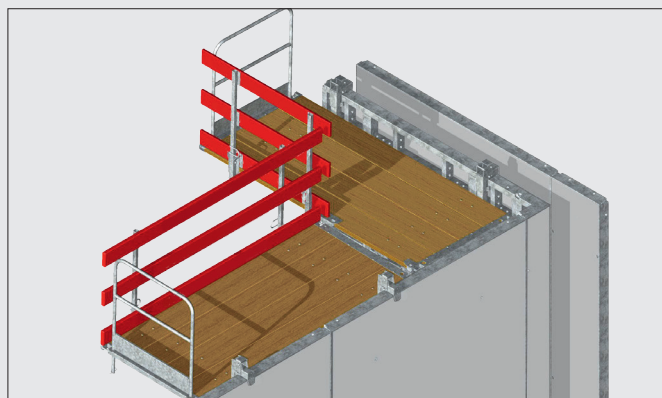
Betonierklappbühne VARIO für Ecklösung mit durchgehender Arbeitsfläche.
